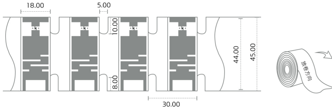
标签结构图
