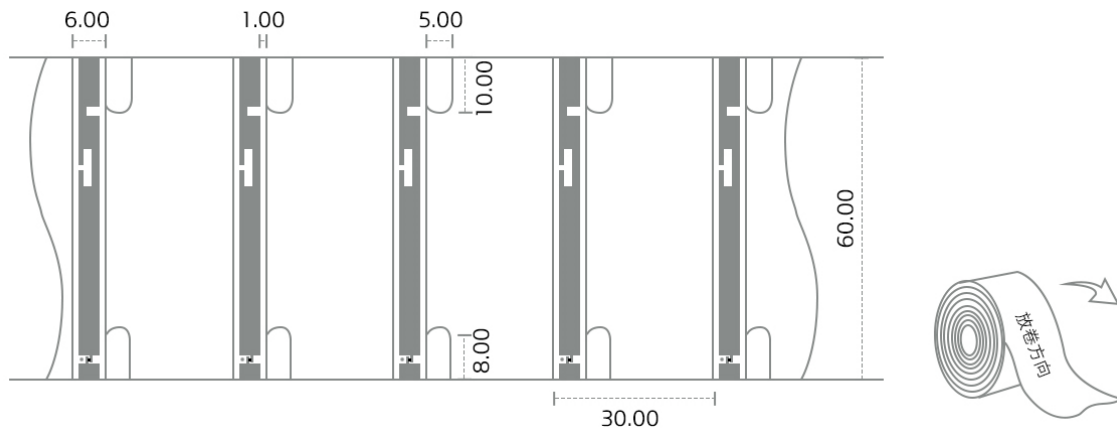
标签结构图
